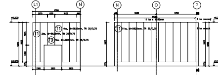
STĚNA „L1“
