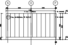
STĚNA „N“
